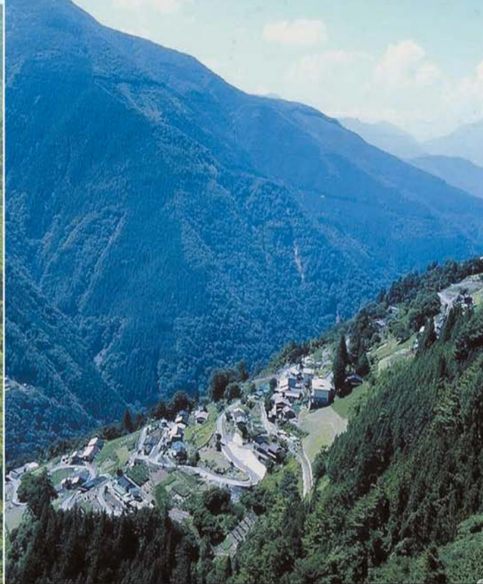
秩父帯の高所集落 (飯田市上村下栗)
