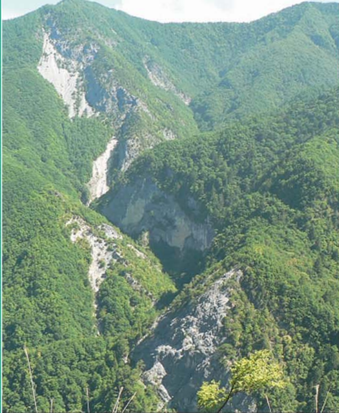
幕岩石灰岩 (伊那市の南アルプス林道からの遠望)
